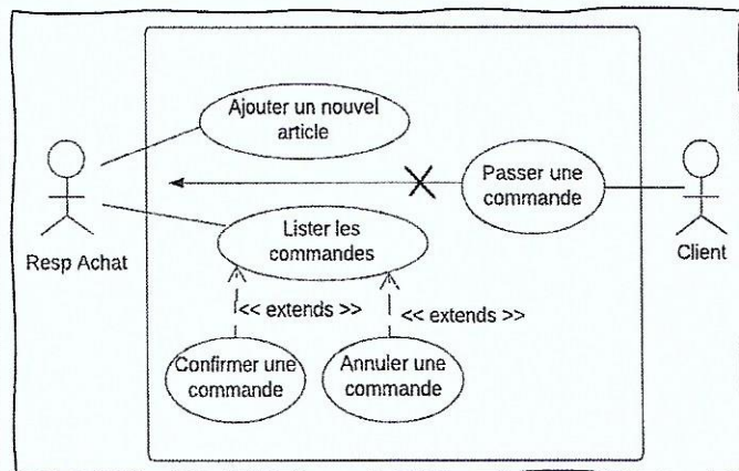
Figure 2 : Interactions entre les utilisateurs et l'application
