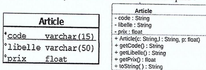
Figure 5 : Modèle relationnel et orienté objet d'un Article
