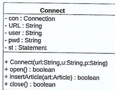
Figure 6 : Classe « Connect »
