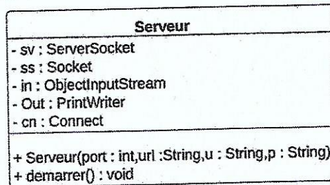
Figure 7 : Classes Serveur
