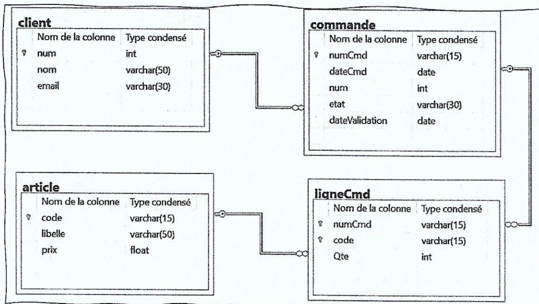
Figure 9 : Modèle logique de données relationnel
