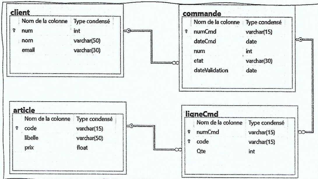
Figure 10 : Partie du Modèle logique de données relationnel
