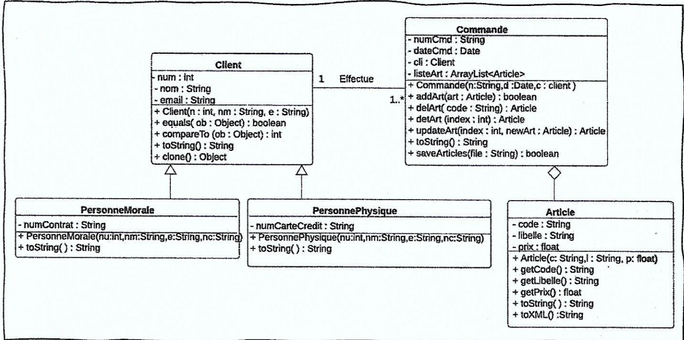
Figure 3 : Diagramme de classes
